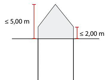
Vooraanzicht dakopbouw met nok haaks op de gevel
