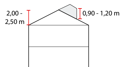
Doorsnede woning met enkelzijdige nokverhoging
