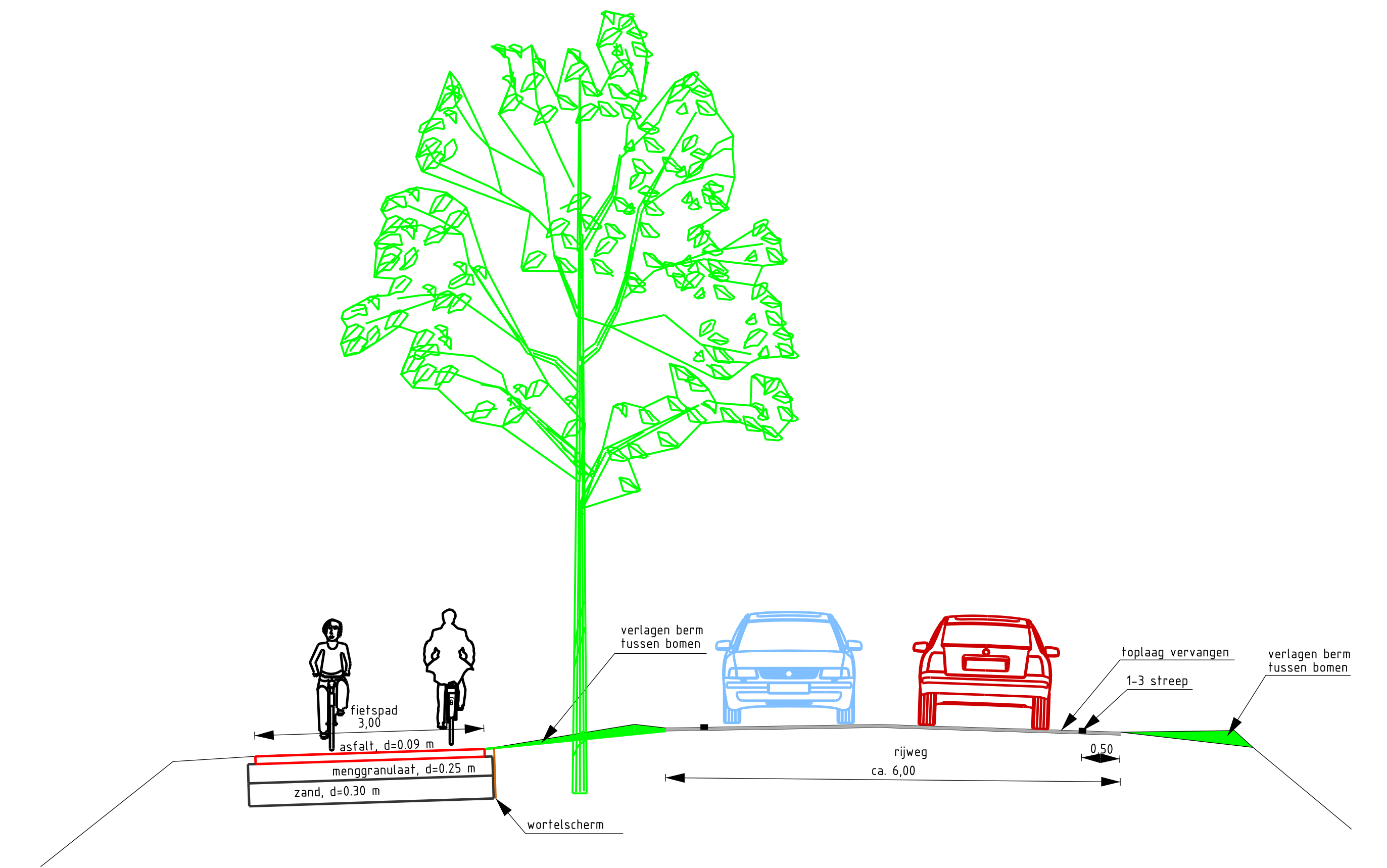
Algemeen dwarsprofiel
