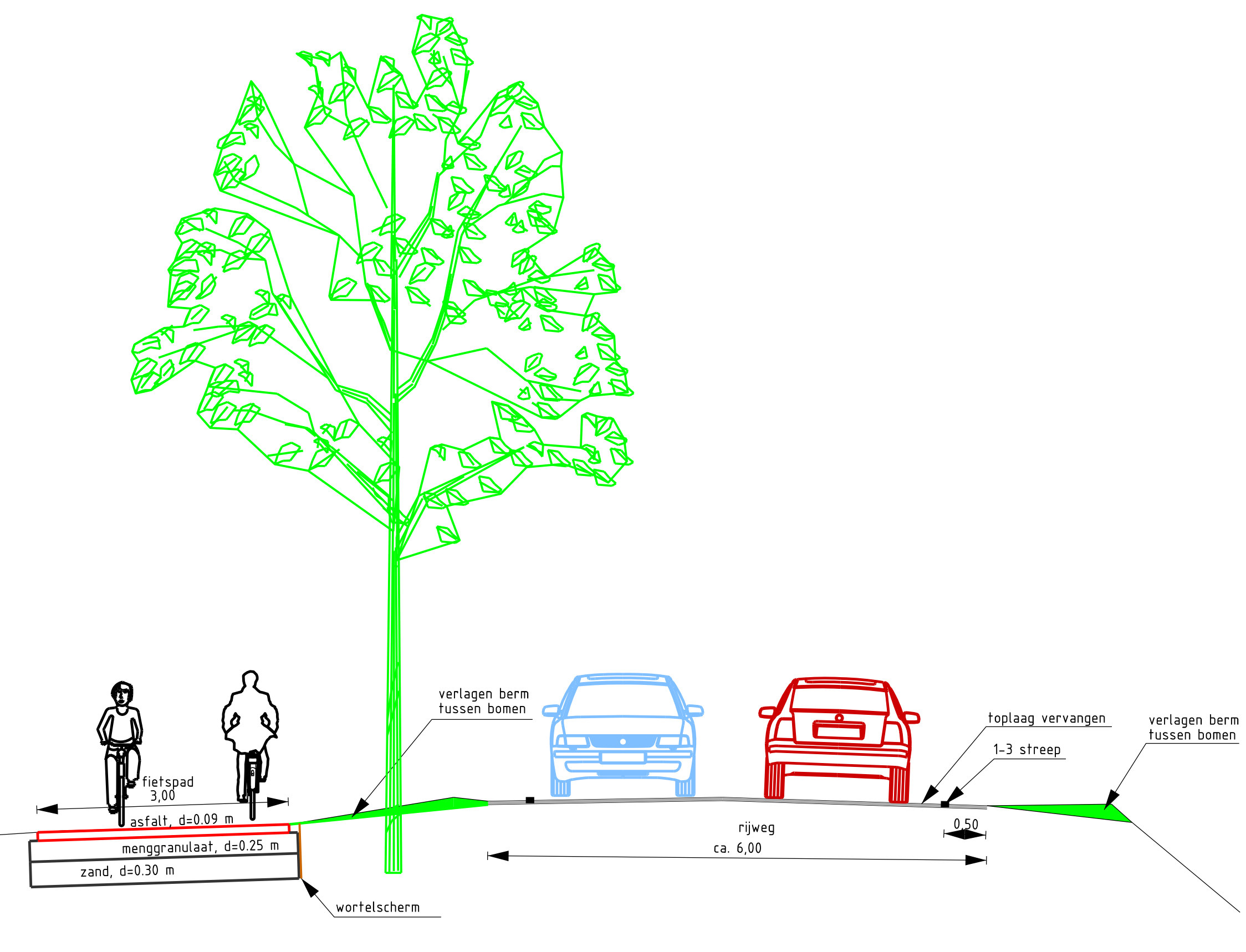
Algemeen dwarsprofiel
