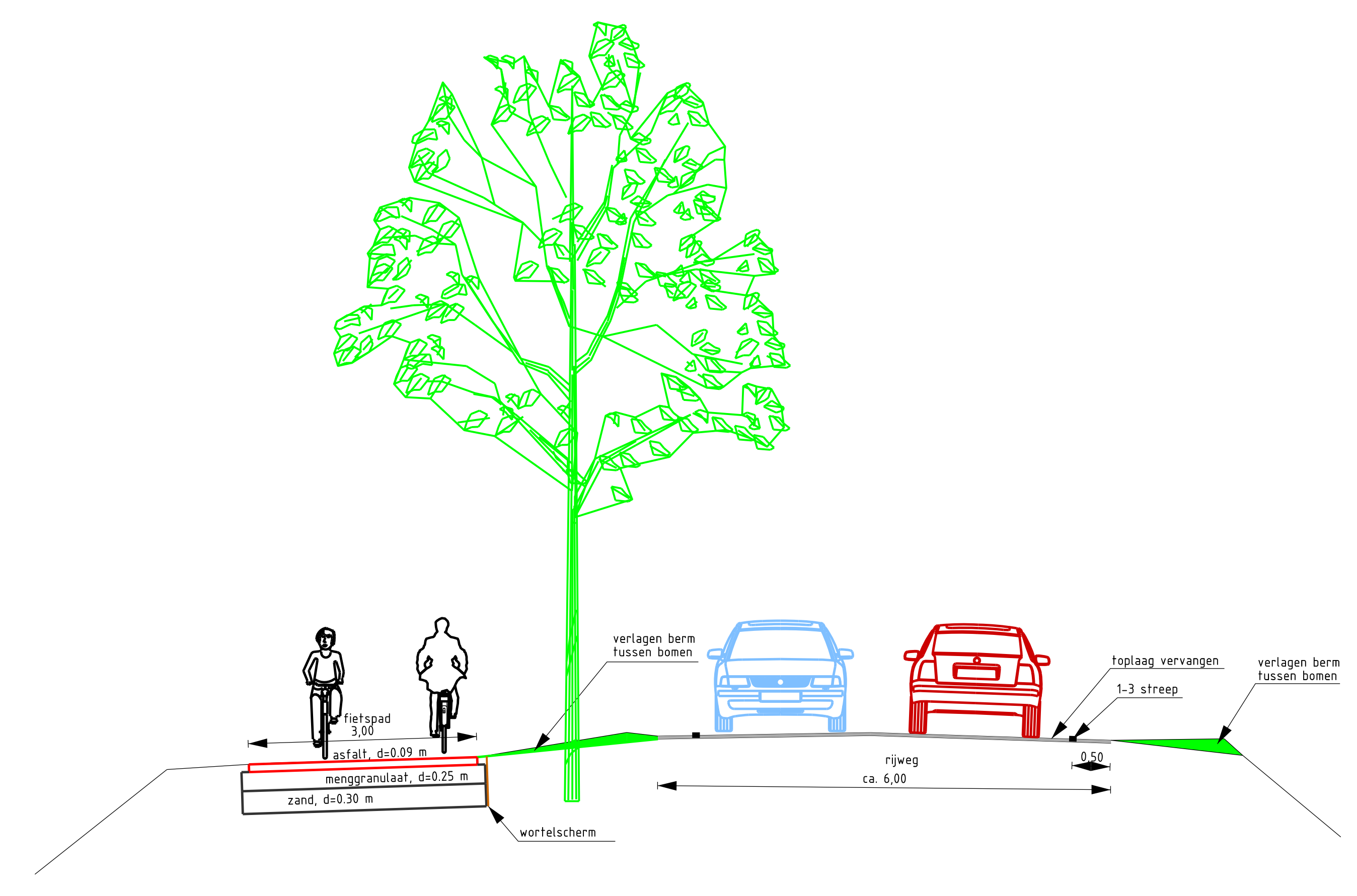
Algemeen dwarsprofiel
