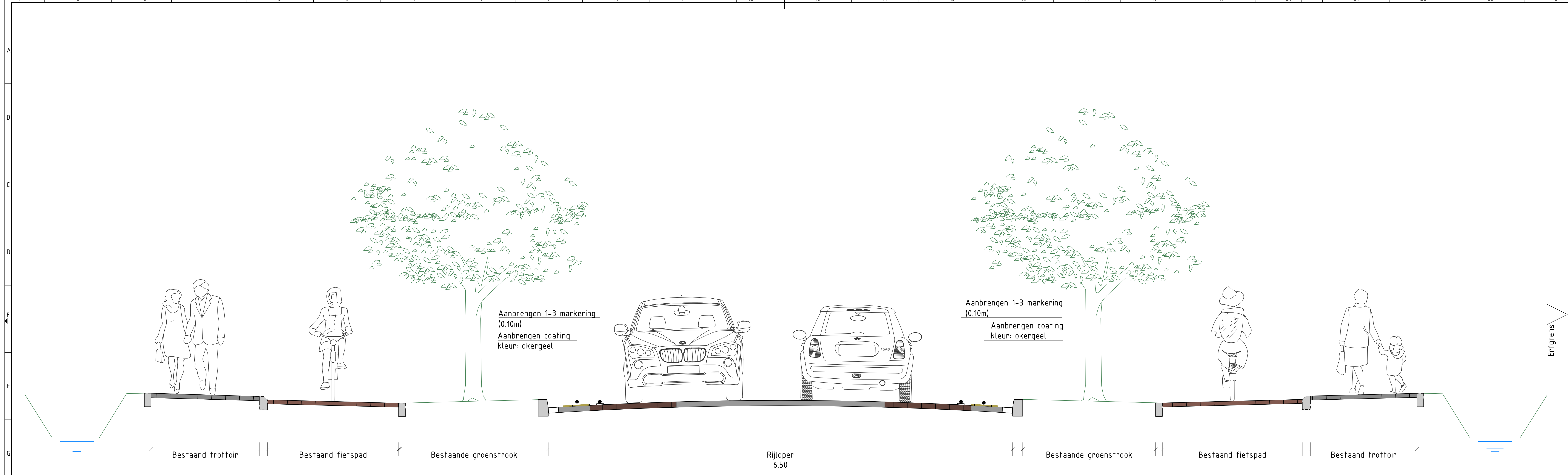
Principe dwarsprofiel 2: Molensingel SCHAAL 1 : 20
