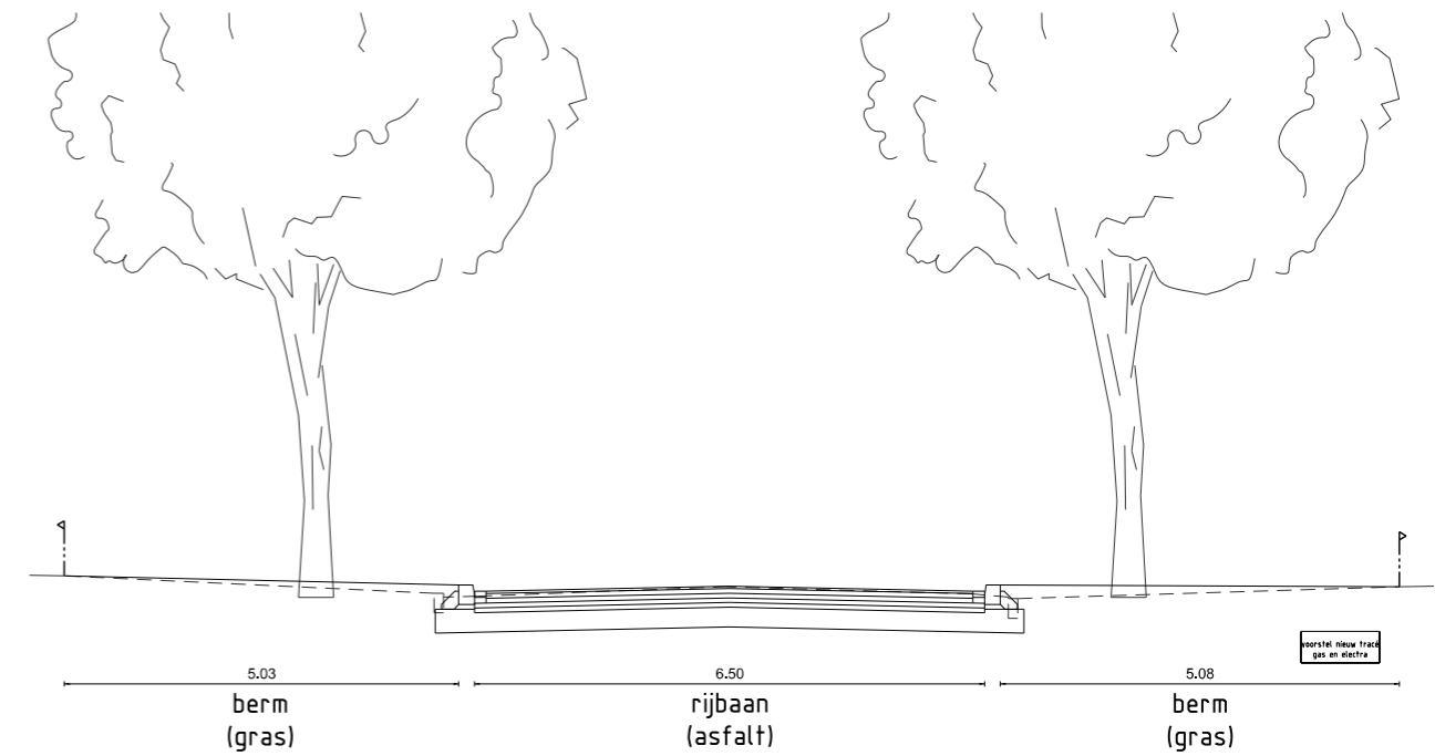
Principeprofiel 1-1
