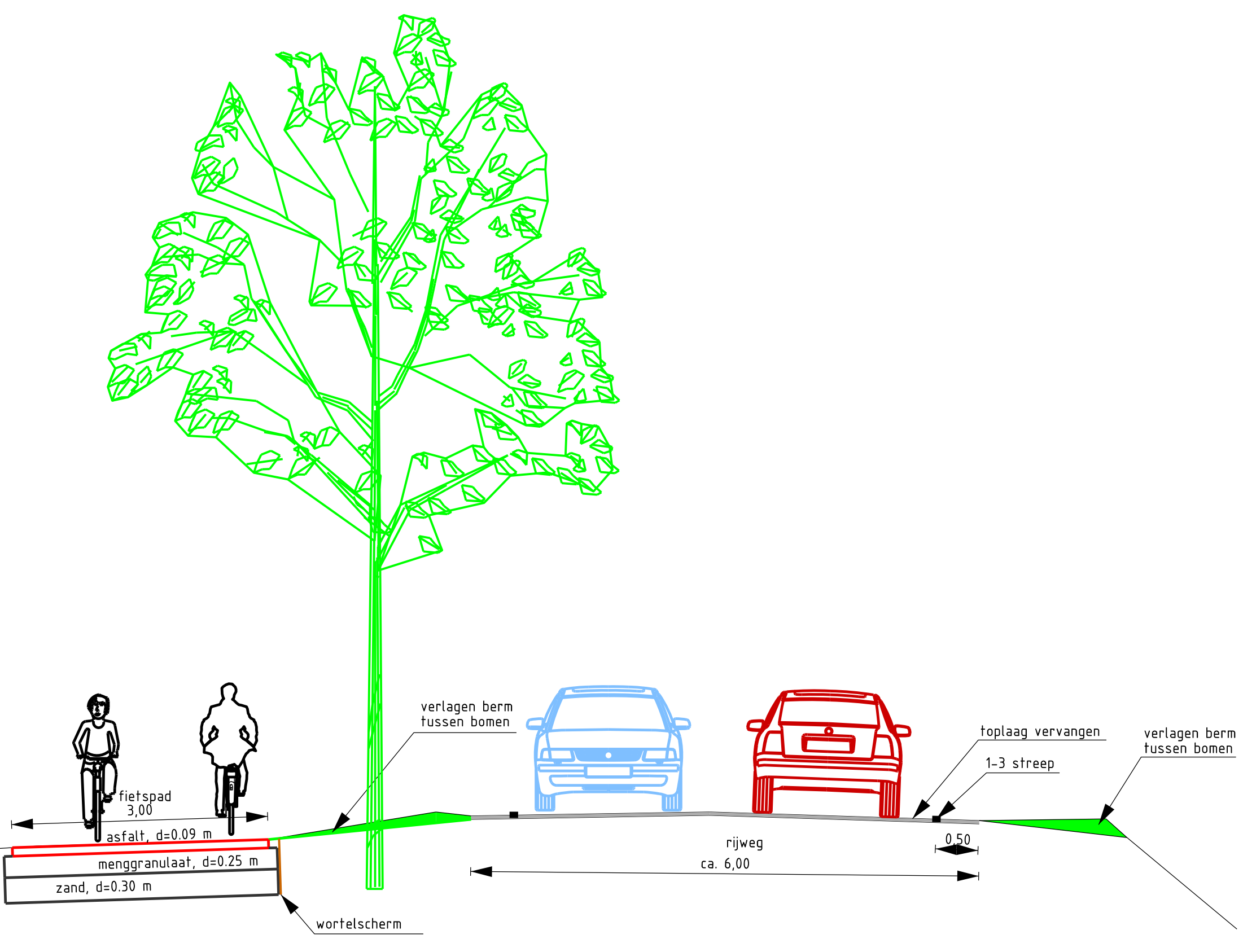
Algemeen dwarsprofiel
