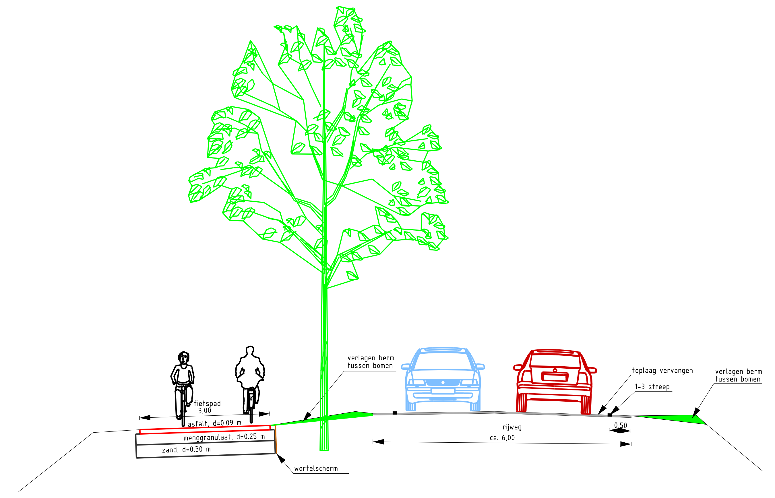
Algemeen dwarsprofiel
