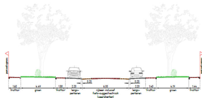
DWARSPROFIEL 1 - ZUIDELIJK DEEL Schaal 1:100
