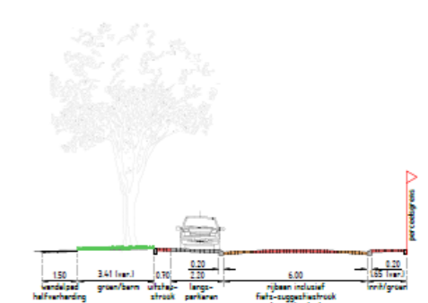
DWARSPROFIEL 2 - NOORDELIJK DEEL Schaal 1:100
