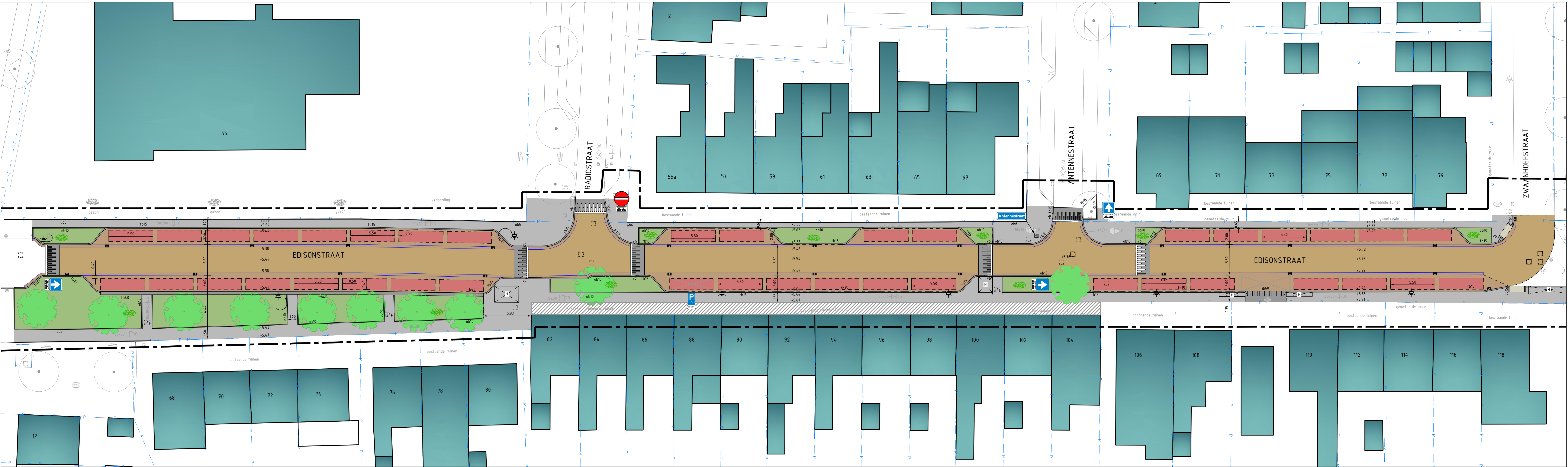
NIEUWE SITUATIE Schaal 1:200
