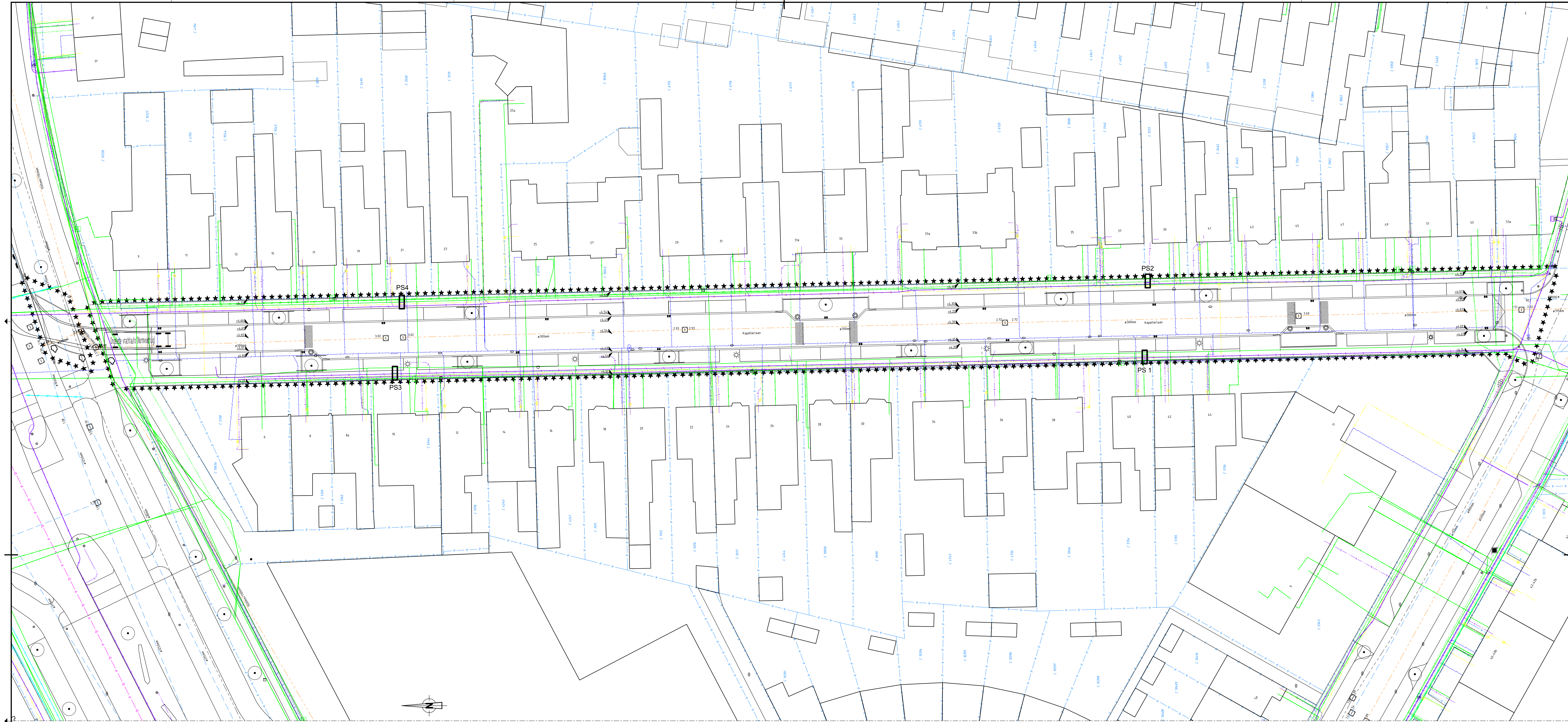
NIEUWE SITUATIE Schaal: 1:200
