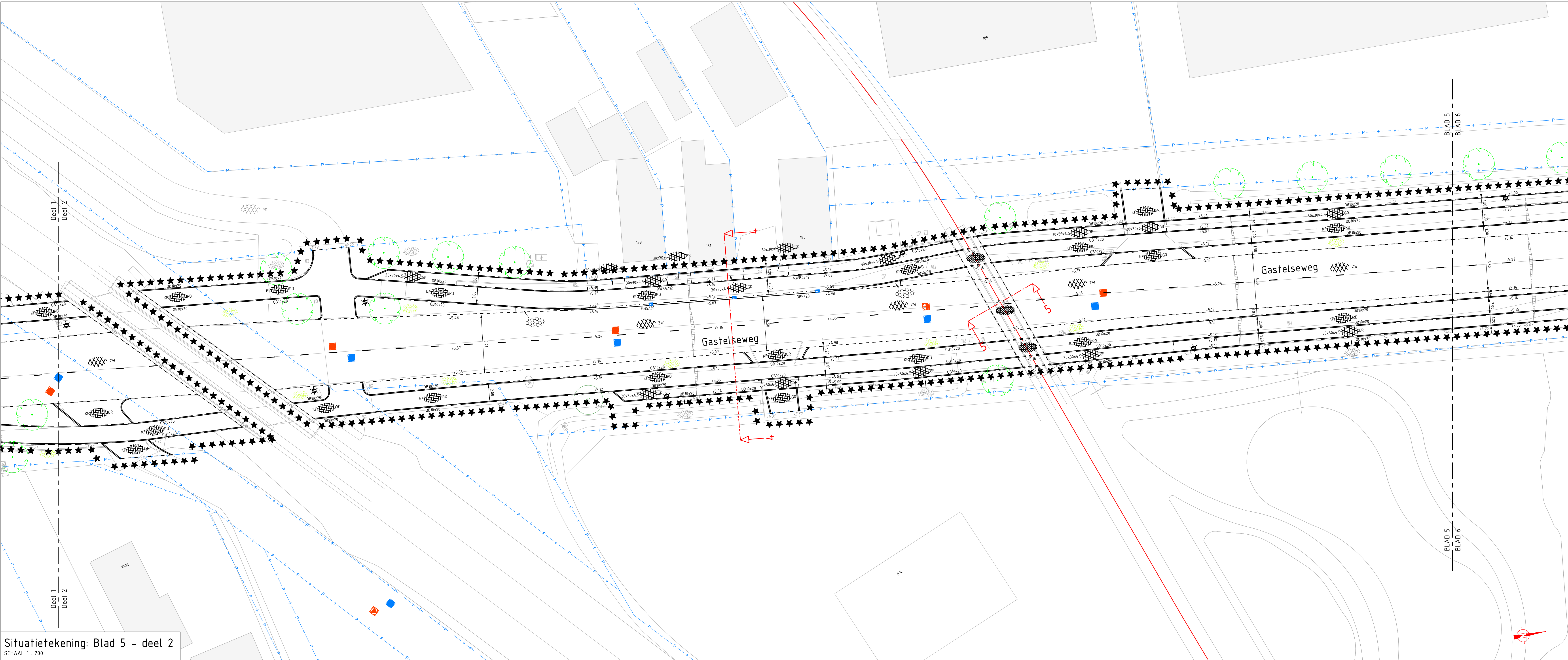
Situatietekening: Blad 5 - deel 1 SCHAAL 1:200
