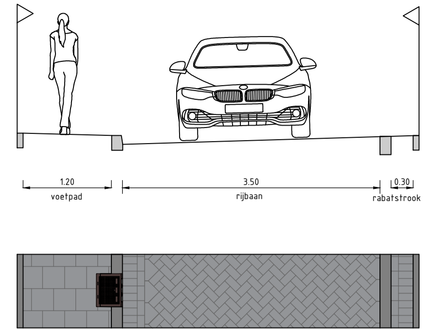
Dwarsdoorsnede 1-1: Dokter Heijpstraat bij P-terrein Schaal: 1:50
