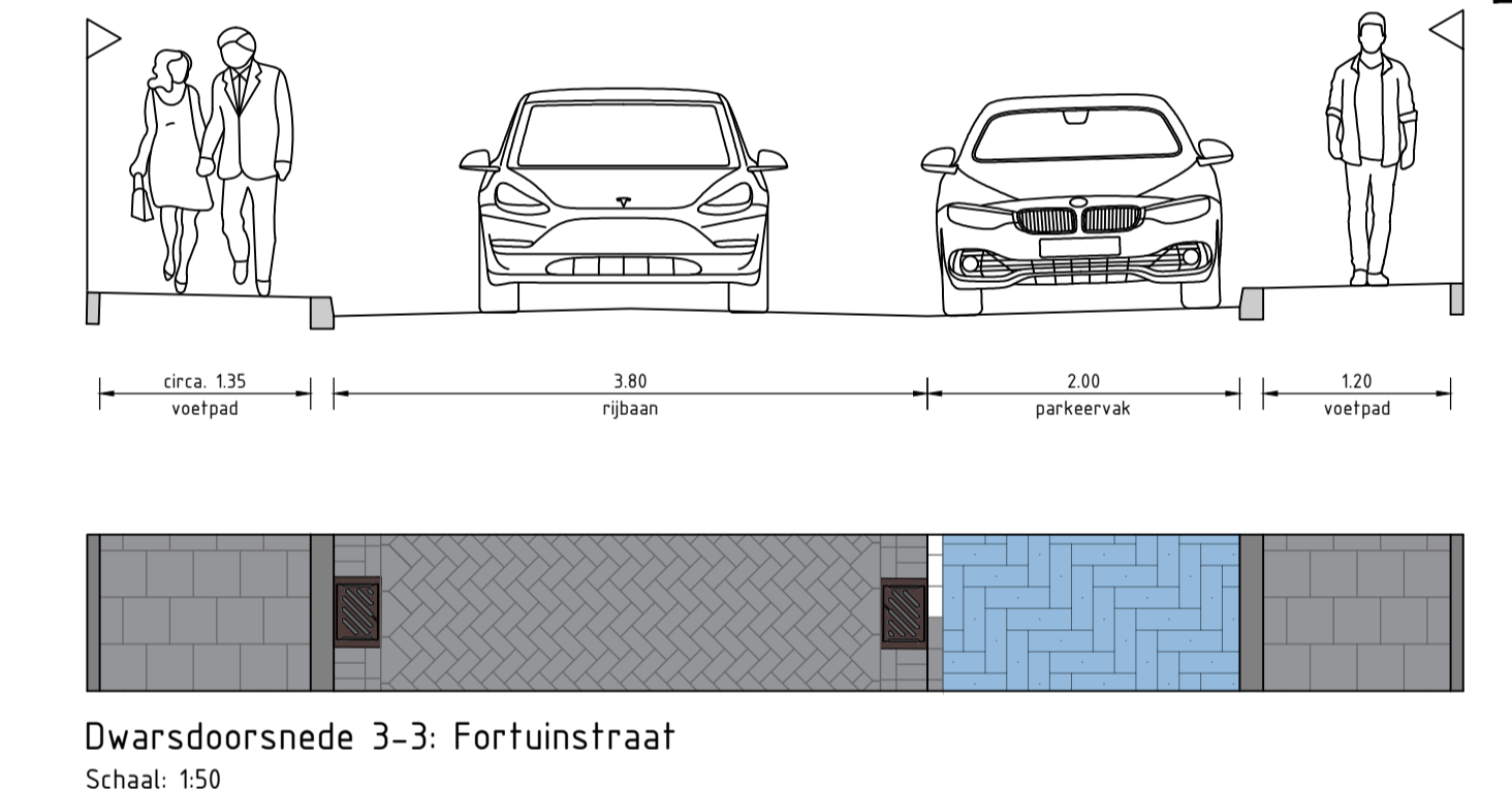
Dwarsdoorsnede 3-3: Fortuinstraat Schaal: 1:50
