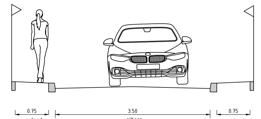
Dwarsdoorsnede 1-1: Dokter Heijpstraat bij P-terrein alternatief Schaal: 1:50
