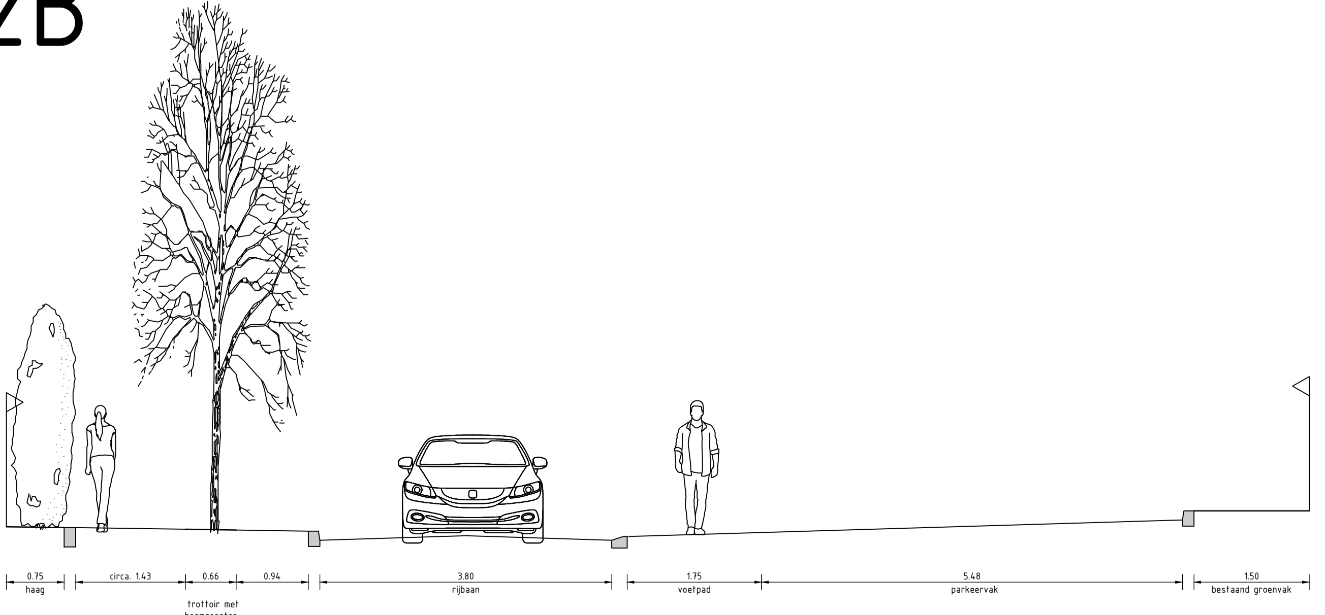
Dwarsdoorsnede 4-4: Dokter Heijpstraat alternatief Schaal: 1:50
