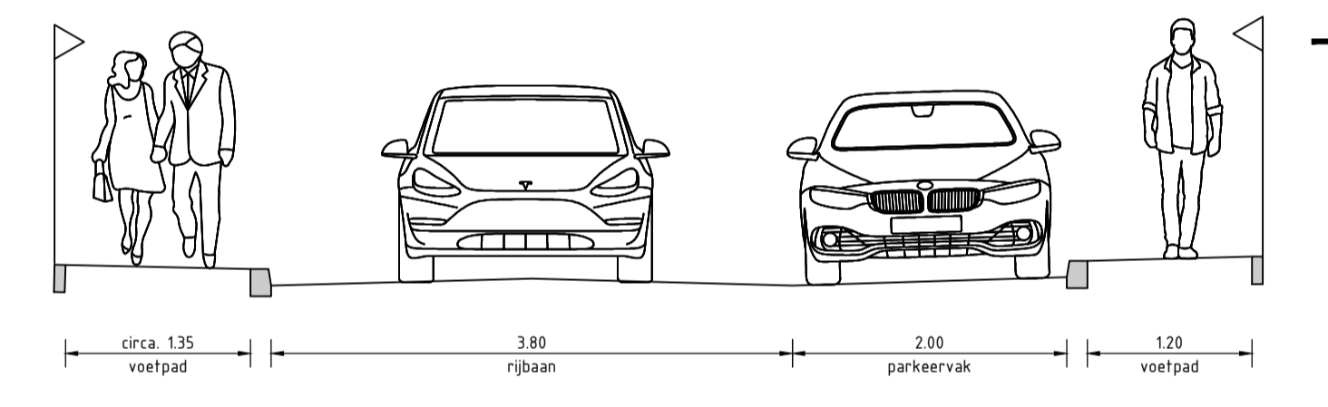
Dwarsdoorsnede 3-3: Fortuinstraat Schaal: 1:50
