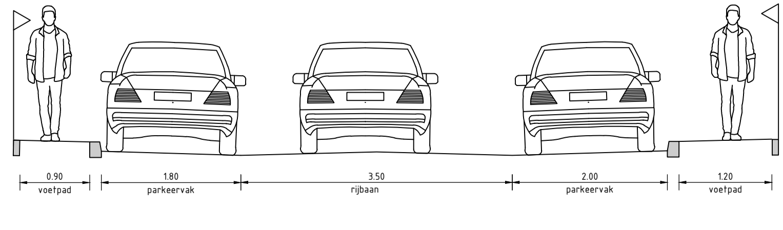
Dwarsdoorsnede 5-5: Fortuinstraat alternatief Schaal: 1:50
